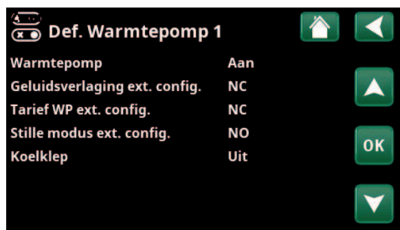
Menu: "Geavanceerd/Definieer/Warmtepomp 1".
