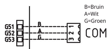
Close-up van bedradingschema.
