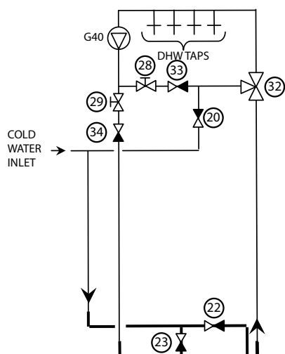
Afbeelding 1 SWW circulatie
