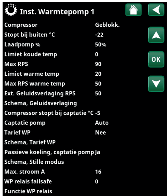
Menu: "Geavanceerd/Instellingen/Warmtepomp/Warmtepomp 1".
