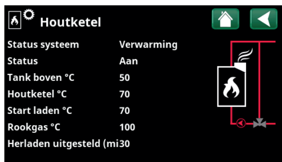
"Werkingsdata/Houtketel" menu.
