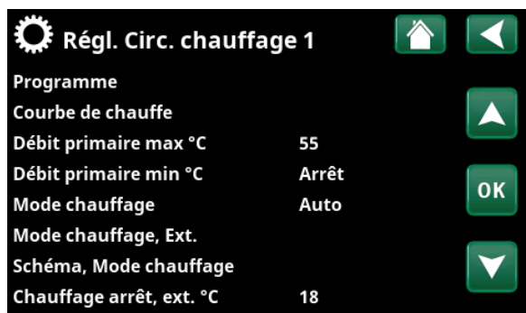
Menu : «Avancé/Réglages/Circ Chauffage». Le mode de contrôle à distance du circuit de chauffage est défini sur la barre de menus «Mode chauffage, externe». Accédez au schéma à partir de la barre de menus «Schéma, Mode chauffage».
