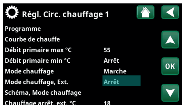
Menu : «Avancé/Réglages/Circ Chauffage/Circ Chauffage 1».
