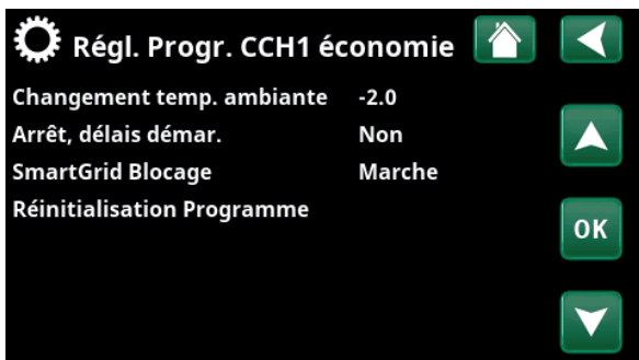
Menu «Avancé/Réglages/Circ Chauffage/Circ Chauffage 1/ Programme/Économie».
