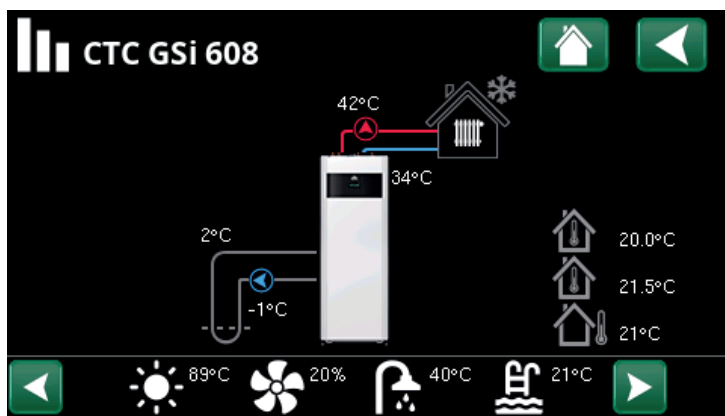
Page de menu principale pour «État opération». Lorsque les pompes sont en fonctionnement, les icônes de pompe tournent sur l'écran.
